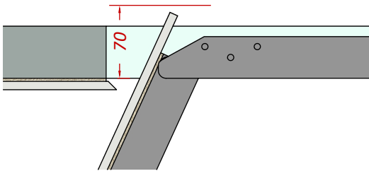
Рис. 3 (вид сверху)
